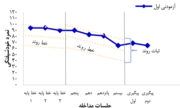
شکل ۷. محفظه ثبات خطوط روند آزمودنی اول
