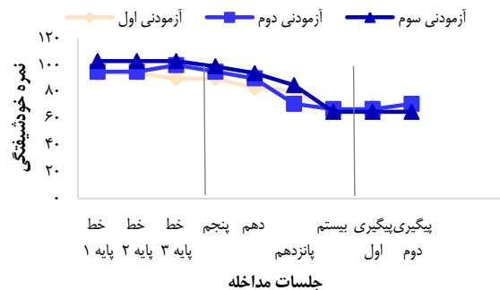
شکل ۵. اثر بخشی طرحواره درمانی بر علایم خودشیفتگی هر سه آزمودنی
