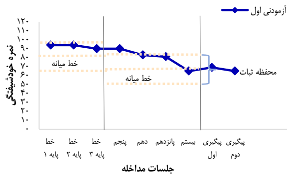
شکل ۶. خط میانه و محفظه ثبات آزمودنی اول
