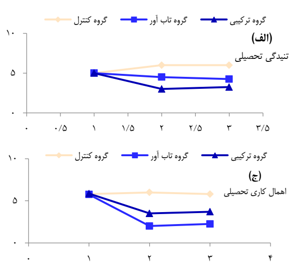
شکل ۱. مقایسه میانگین‌های برآورد حاشیه‌ای گروه‌های تاب‌آور، ترکیبی و شاهد در مراحل پیش‌آزمون، پس‌آزمون و پیگیری در هر چهار متغیر وابسته
