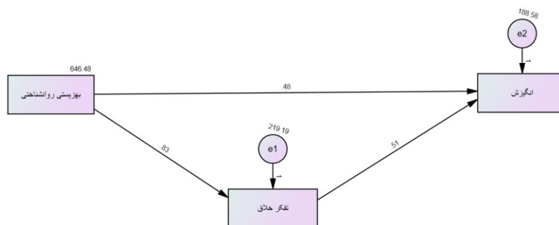
نمودار ۱: ضرایب غیراستاندارد مدل مورد مطالعه
