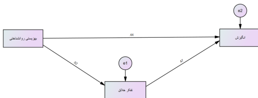
نمودار ۲: ضرایب استاندارد مدل مورد مطالعه
