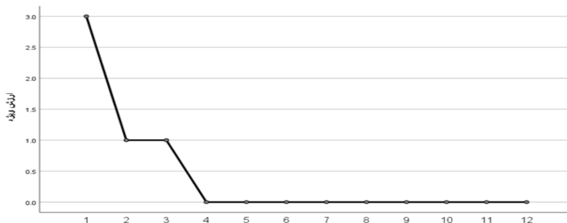
نمودار ۱. نمودار سنگ ریزه در تحلیل عامل‌ها
