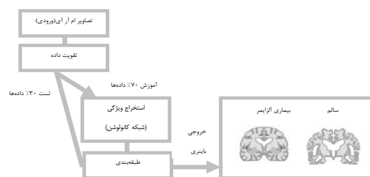
شکل ۳. نمایشی از چارچوب پیشنهادی
