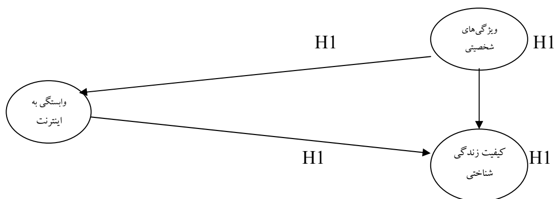
نمودار ۱. مدل نظری پژوهش بر مبنای Yang (۶)
